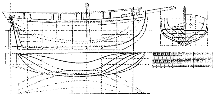
Skisse av Peter N. Søllings plattgattede båt «Rosenkrantz». + Gothe Gøthesen: Norske Båter. B. 1 – Skagerakkysten. Oslo 1977.
