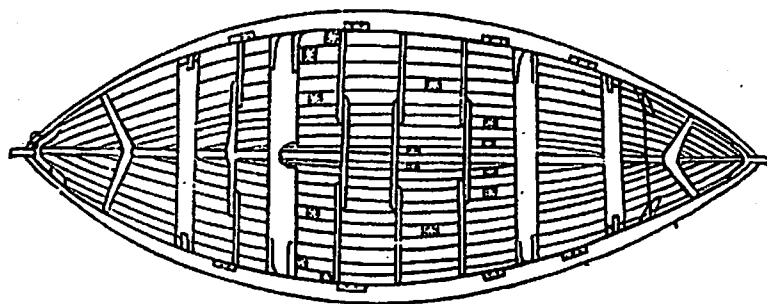
Åpen, spririgget listerbåt. + Tegnet av Eilert Sundt.
